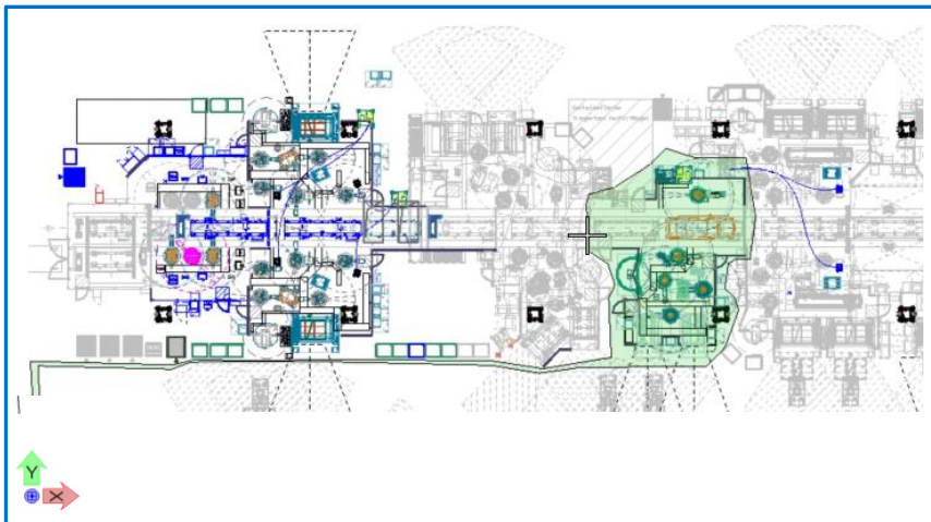
Gesamt-Layout
